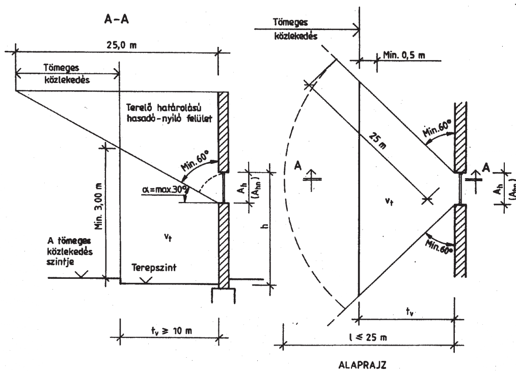
5. ábra, A lefúvás környezetének védelme alcímhez
