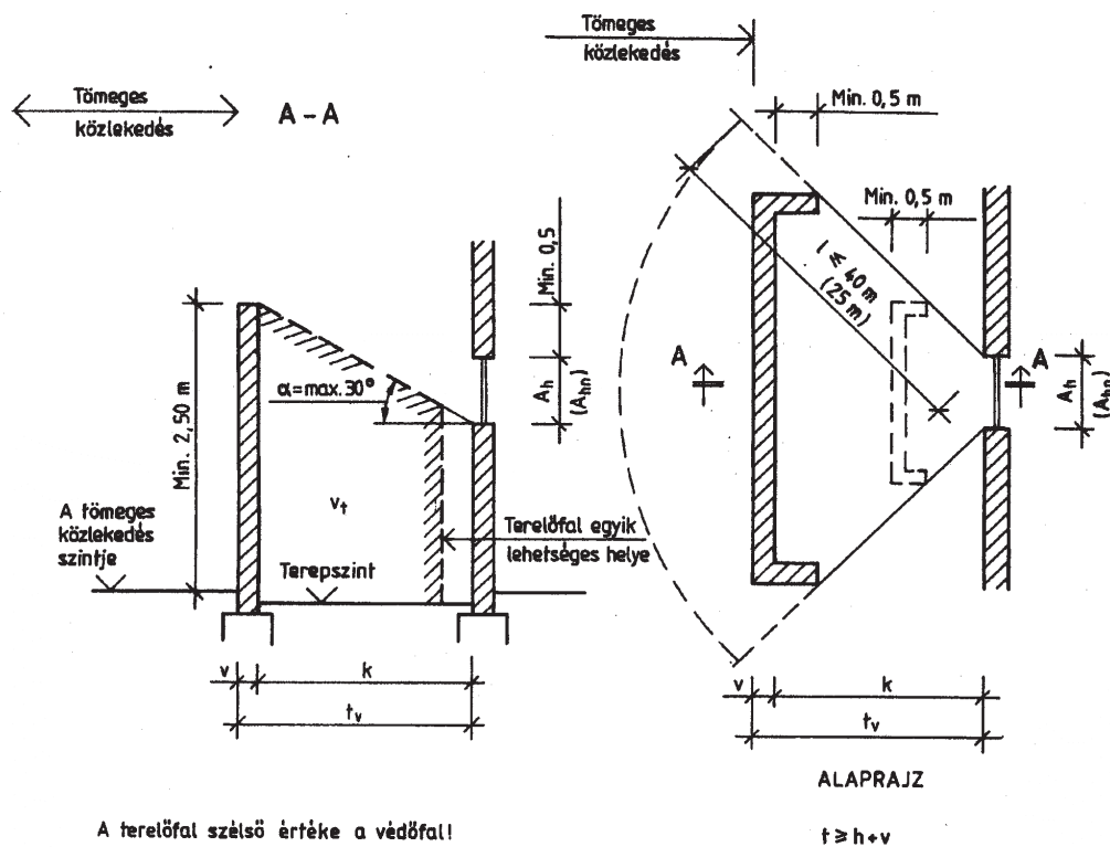
5. ábra, A lefúvás környezetének védelme alcímhez
