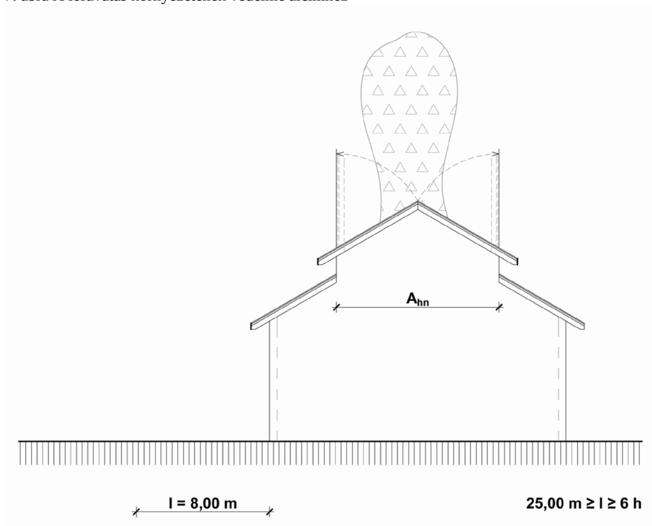
7. ábra A lefúvatás környezetének védelme alcímhez
