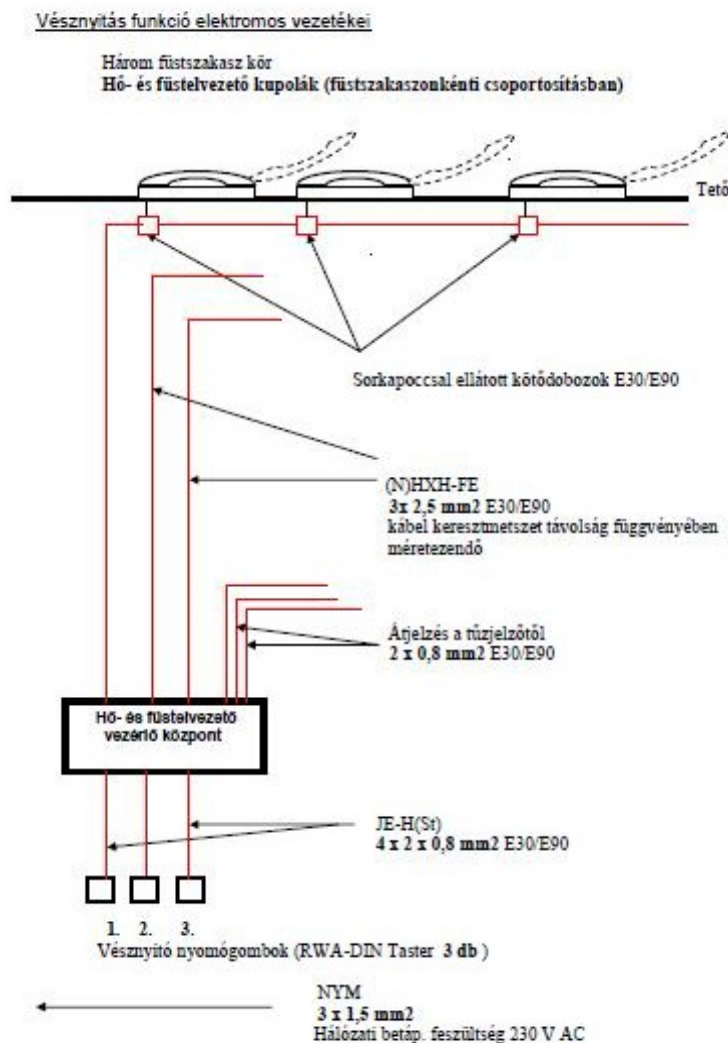
3. ábra: Automatikus (tűzjelző érzékelő általi) vésznyítás megoldásának példája
