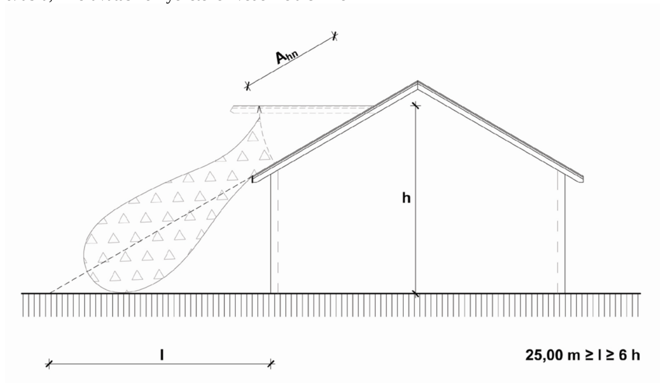
6. ábra, A lefúvatás környezetének védelme alcímhez
