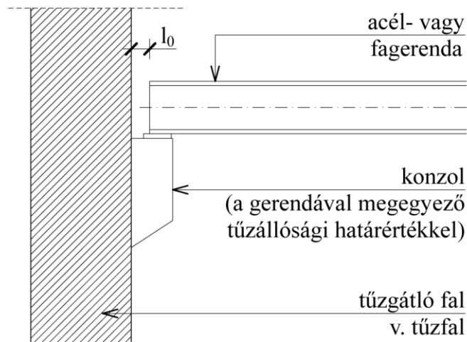
15.5 sz. ábra. Tűzgátló fal és tűzfal elválasztása kedvezőtlenebb tűzvédelmi jellemzőjű építményszerkezetektől
