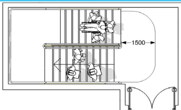
14. ábra: Kerekessel történő mentésre alkalmas lépcsőház minimális méretei
