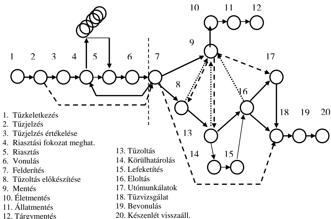
7. ábra. A tűzoltás folyamata a Tűzoltási Szabályzat pontjai alapján. Forrás: Szerző.
