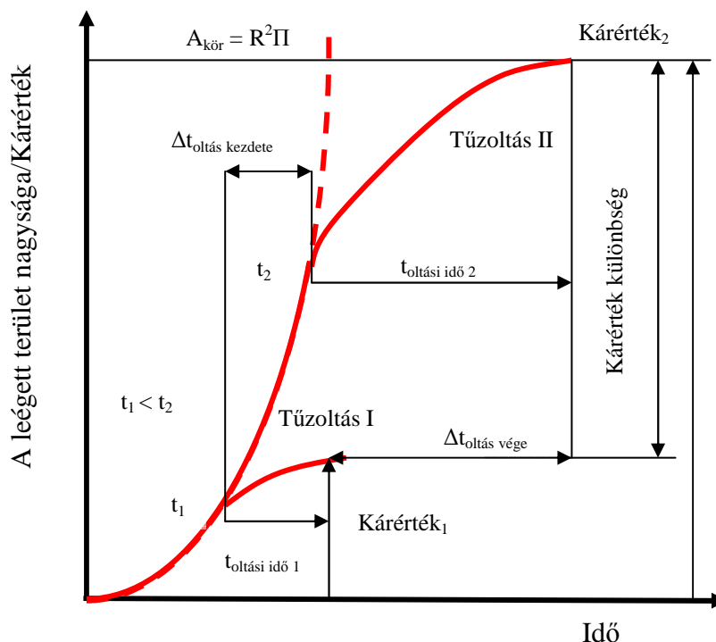
3. ábra. Kárérték–Idő függvény erdőtüzre vonatkoztatva. Forrás: Szerző.
