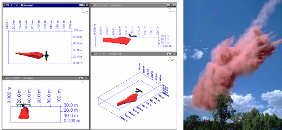
28. ábra. Az oltóanyag kibocsátásának vizsgálata több metszetben. Forrás: Tomé.
