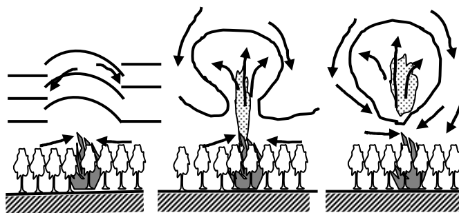
13. ábra. A buborék kialakulásának fázisai.
