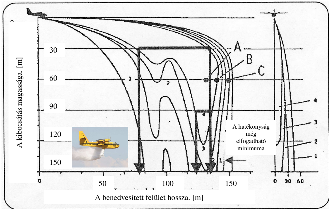
46. ábra. Az egységnyi felületre jutó oltóanyag mennyisége a reológiai görbék segítségével és a repülési magasság függvényében. Forrás: Hardy, C. nyomán a Szerző.
