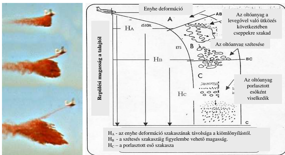
26. ábra. Az oltóanyag viselkedése a kibocsátás után. Forrás: Hardy.
