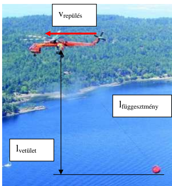
34. ábra. A függesztmény vetülete üres tartály esetén. Forrás: a kép alapján a Szerző.
