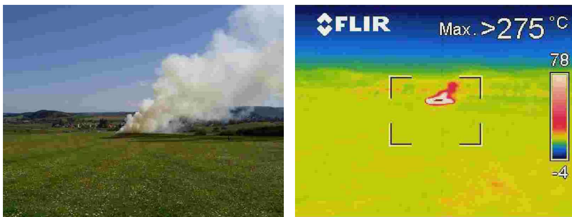
15. kép Kísérleti tűz vizuális és hőképe. Forrás: Szerző magánarchívuma.
