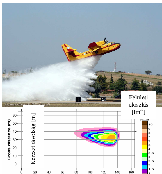
32. ábra. Az oltóanyag felületi eloszlása. Forrás: Tomé.
