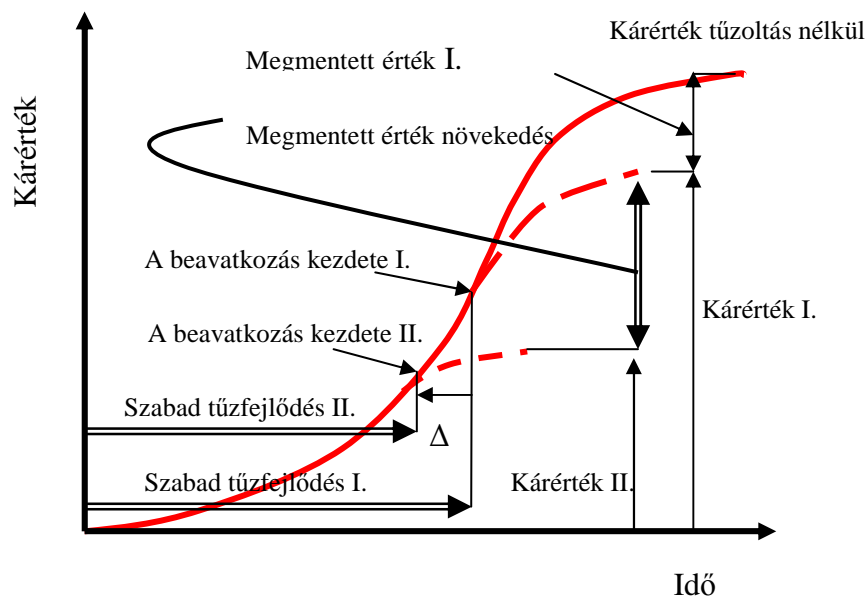
2. ábra. Kárérték–Idő függvény különböző riasztási időpontokra vonatkoztatva. Kárérték az oltás megkezdésének függvényében. Forrás: Bleszity nyomán a Szerzőtől.
