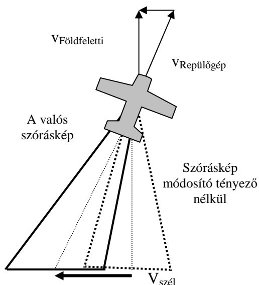
42. ábra. A szóráskép elmozdulása a szél hatására. Forrás: Szerző.
