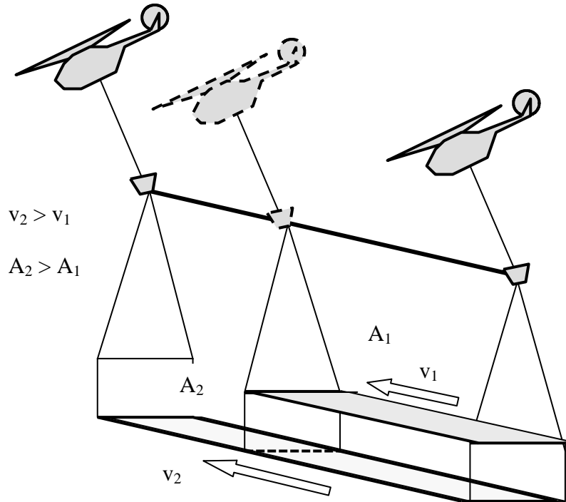
39. ábra. A repülési sebesség változásának hatása a szórt felület nagyságára. Forrás: Szerző.
