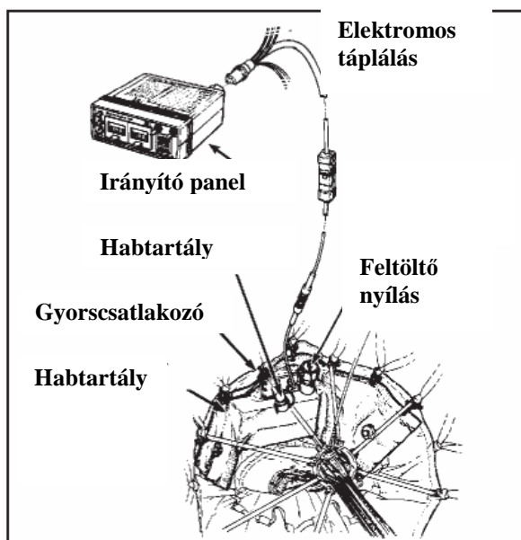
10. ábra. Sacksafoam rendszer vázolata. Forrás: Internet.
