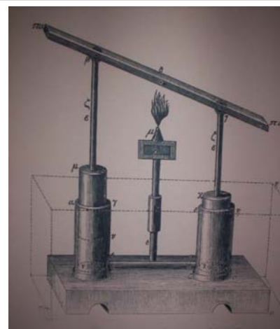
33. kép. Héron által tökéletesített szivattyú elvi rajza
