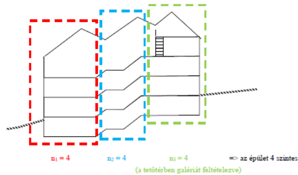
1. ábra: Példa szinteltolásokos lakóépület szintszámának megállapítására
