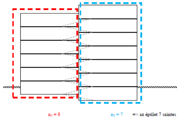
2. ábra: Példa félszinteltolásokos gépjárműtároló szintszámának megállapítására
