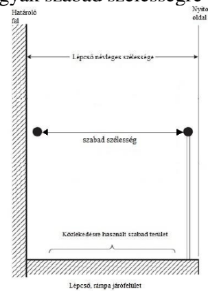
C6. ábra: Lépcsők, rámpák szabad szélessége
