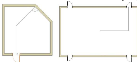
C2. ábra: Példák a kiürítési út hosszának megállapításár
