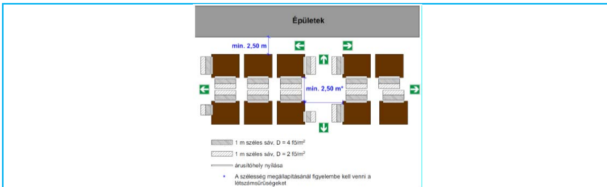
3. ábra: a létszámsűrűségek meghatározása
