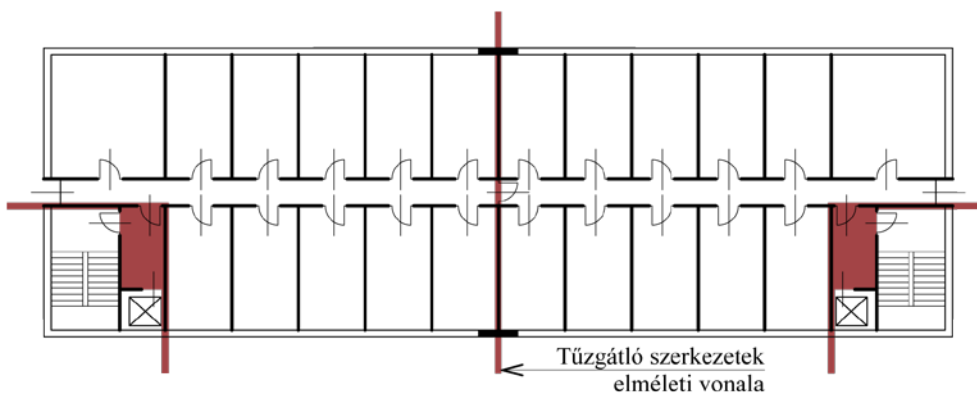
F3. ábra Függőleges tűzszakasz-határral szintenként két tűzszakaszra osztott épületrész, két átmeneti védett tér és lépcsőház együttesével, mindkét oldalon menekülési felvonóval F4. A lépcsőház pihenőjének, illetve előterének átmeneti védett térként történő javasolt kialakítási lehetőségei
