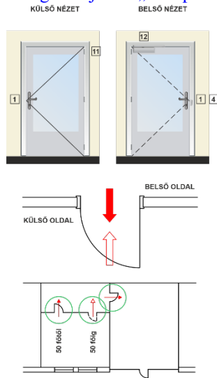
JELMAGYARÁZAT 1 - kilincs 4 - cylinder betétes bevésőzár tűzgátló ajtónál: 11 - rugós pántba rejtett ajtócsukó, vagy 12 - sínes / karos (tűzgátló) ajtócsukó
