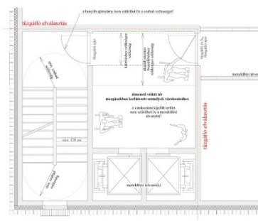
F3. ábra Függőleges tűzszakasz-határral szintenként két tűzszakaszra osztott épületrész, két átmeneti védett tér és lépcsőház együttesével, mindkét oldalon menekülési felvonóval F4. A lépcsőház pihenőjének, illetve előterének átmeneti védett térként történő javasolt kialakítási lehetőségei
