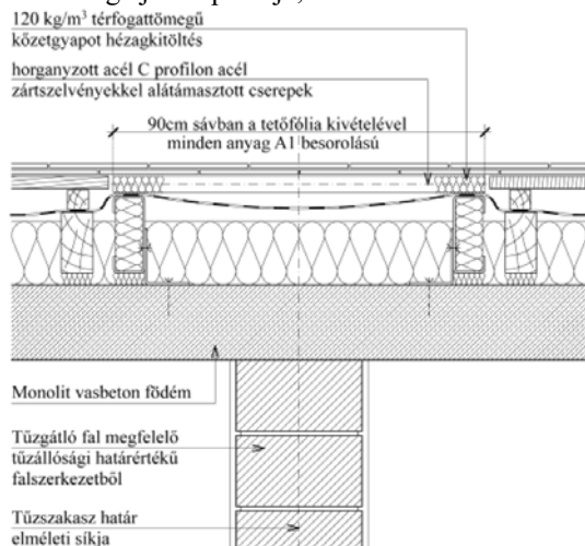
F4 sz. ábra: magastető tetősíkból kiemelkedő tetőszinti tűzterjedés elleni gátja kialakításának példája, vasbeton koporsófödém esetén
