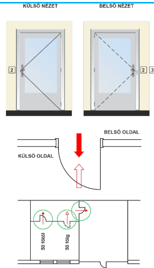
JELMAGYARÁZAT 2 - húzórud vagy fogógomb, rugós zárnyelv 3 - cylinder betét nélküli bevésőzár
