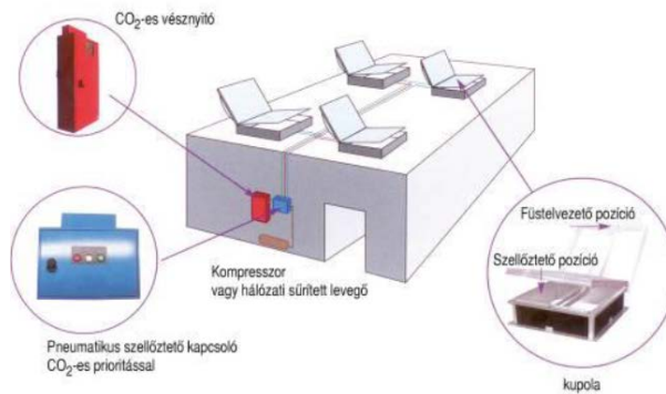
12. ábra: Példa munkahengeres vésznyitás és munkahengeres szellőztetés megoldására
