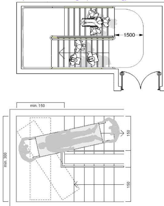
14. ábra: 2Kerekesszékkel és hordágyal történő mentésre alkalmas lépcsőház minimális méretei
