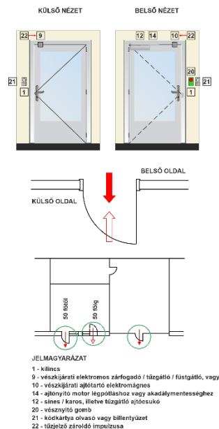
G20. ábra: Egyszárnyú, elektromos zárassal rendelkező homlokzati ajtók / tűzgátló vagy légpótló ajtók – „D” típus
