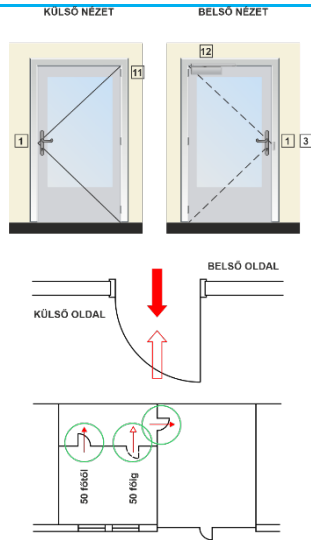
JELMAGYARÁZAT 1 - kilincs 3 - cylinder betét nélküli bevésőzár 11 - rugós pántba rejtett ajtócsukó, vagy 12 - sínes / karos, illetve tűzgátló ajtócsukó
