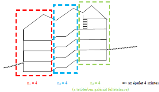
1. ábra: Példa szinteltolások lakóépület szintszámának megállapítására
