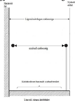
C6. ábra: Lépcsők, rámpák szabad szélessége
