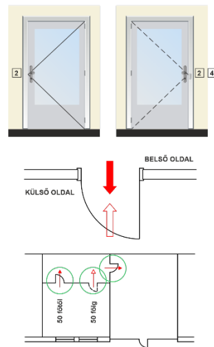
JELMAGYARÁZAT 2 - húzórud vagy fogógomb, rugós zárnyelv 3 - cylinder betétes bevésőzár
