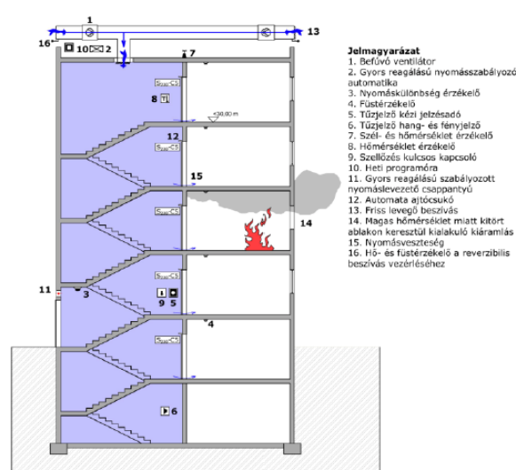
H-4. ábra: Példa túlnyomásos füstmentes lépcsőház tetőszintű frisslevegő beszívásának lehetőségére
