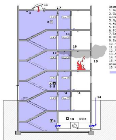
H-2. ábra: Példa előteres túlnyomásos füstmentes lépcsőház kialakítására, szabályozott üzemi ventilátorral, túlnyomás leveztető kupolával
