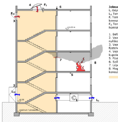
H-1. ábra: Példa a természetes hő- és füstelvezetéssel ellátott lépcsőház kialakítására különböző léghajtási variációkkal
